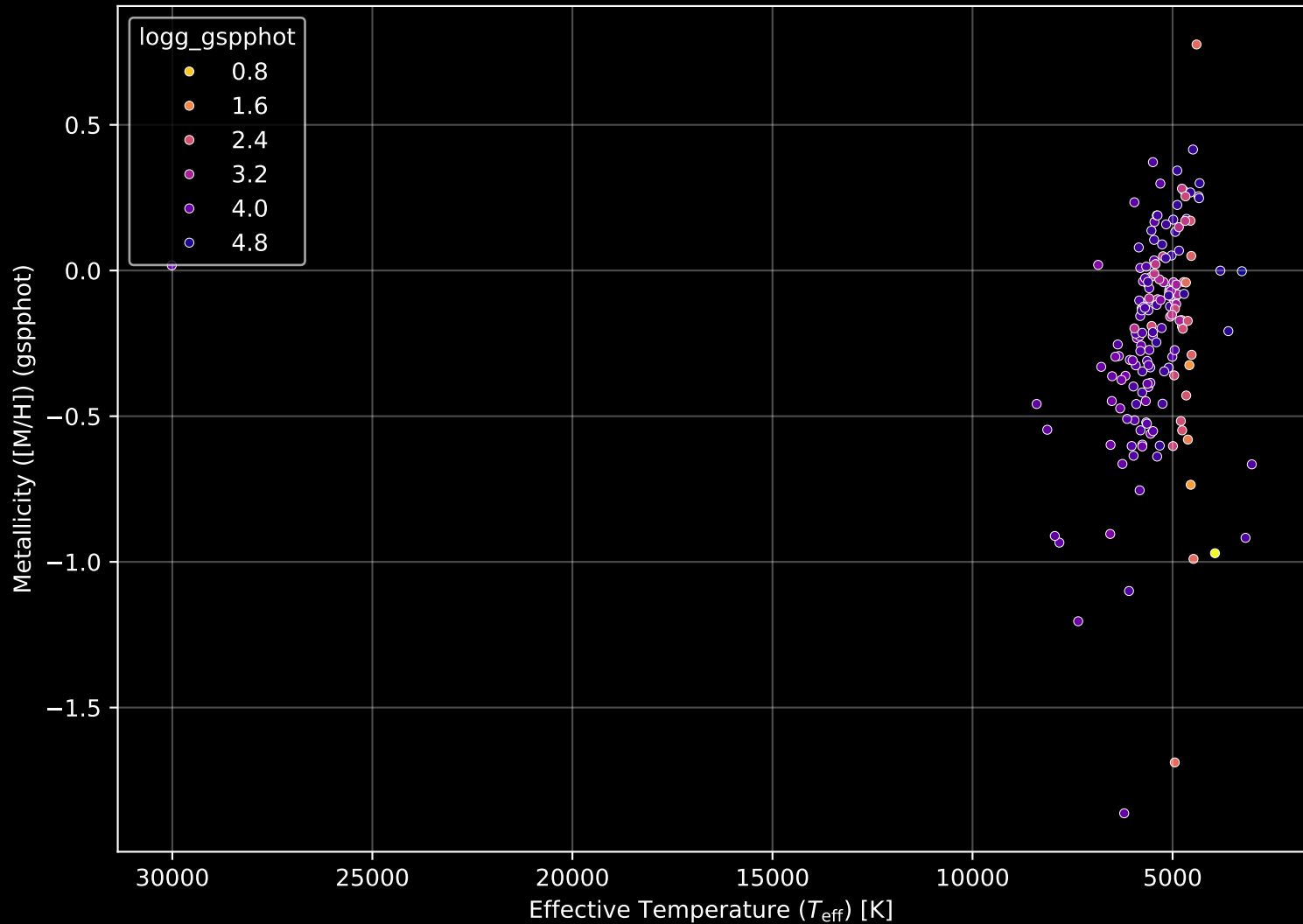
APOGEE DR17 Field: [284-30-O_TESS] Stellar Population Parameters (n= 169)
