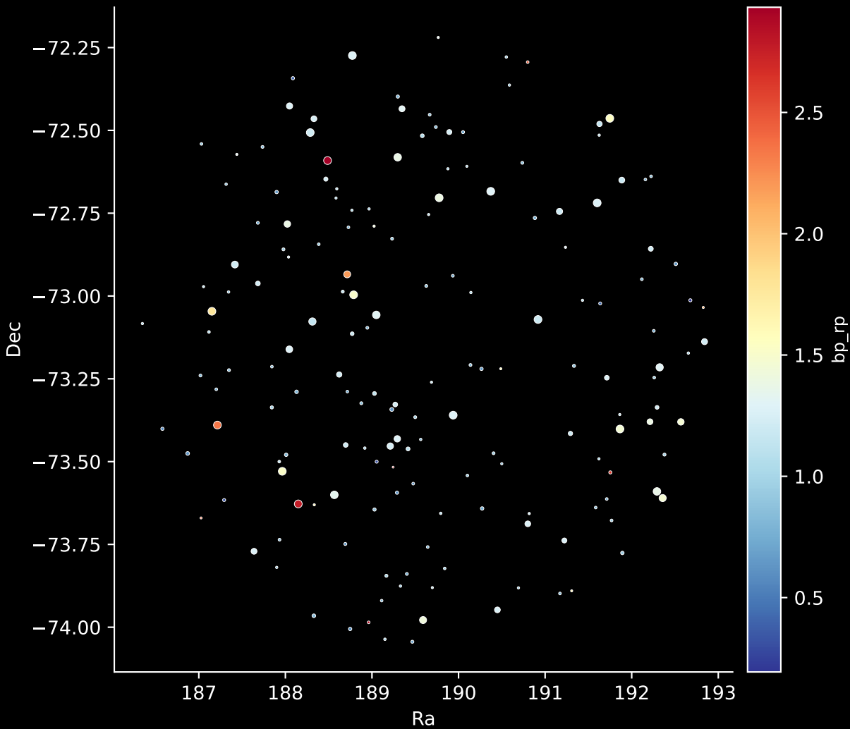
APOGEE DR17 Field: [284-30-O_TESS] Stars: 169
